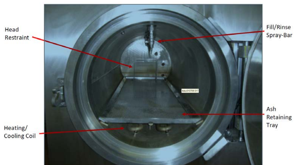
Figuur 4 Binnenkant van de resomator [5]
