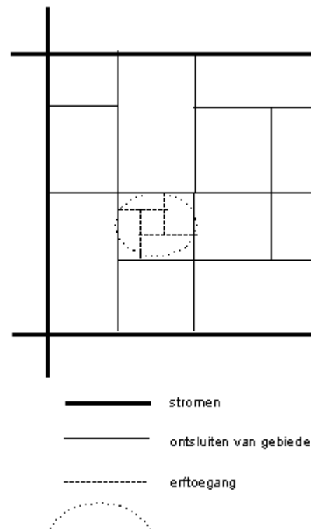
Figuur 1 schematisch overzicht van functies in een duurzaam veilig wegennet
